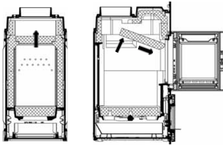
Abb. 3.8 Entnehmen der Umlenkung
