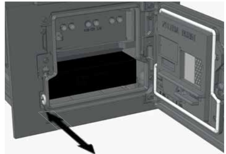
Abb. 3.3 Rüttelstange für die Rosteinrichtung, links unten neben dem Aschefach (rechts angeschlagene Aschefachtür)
