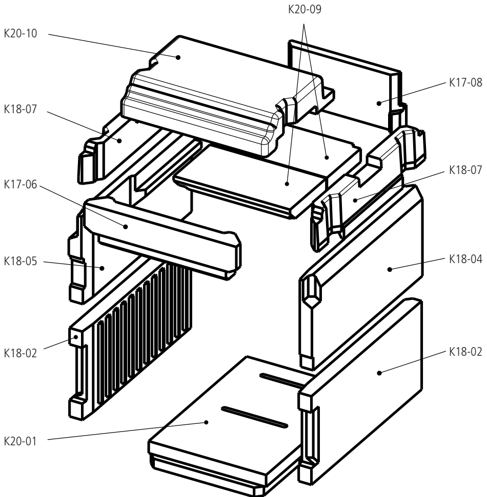
Abb. 7.4 Feuerraumauskleidung RUBIN K20
