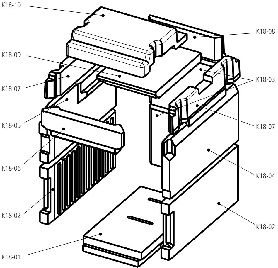
Abb. 7.2 Feuerraumauskleidung RUBIN K18
