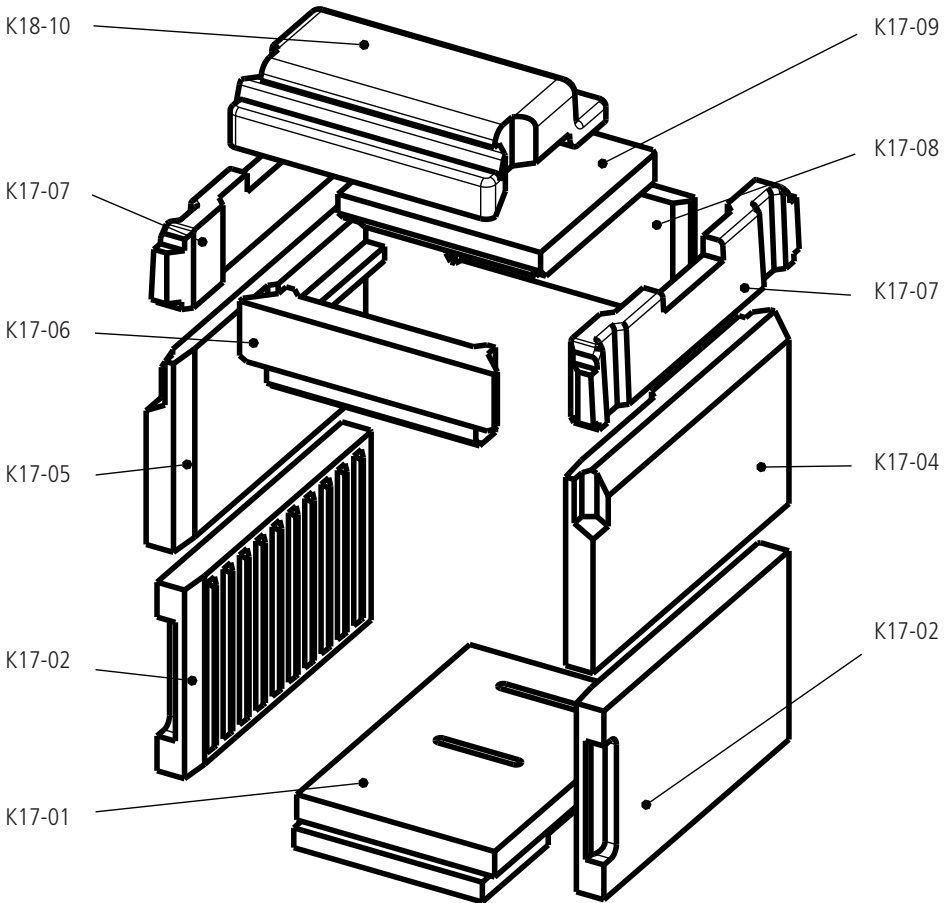
Abb. 7.1 Feuerraumauskleidung RUBIN K16 und K17
