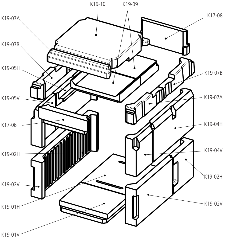
Abb. 7.3 Feuerraumauskleidung RUBIN K19
