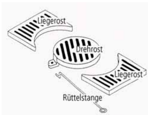
Abb. 7.5 Ersatz- und Verschleißteile, Rosteinrichtung RUBIN
