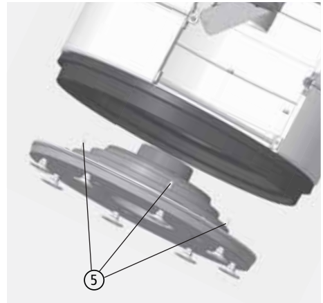
Abb. 3.22 Drehkonsole unter dem COLONA befestigen
