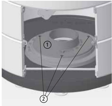
Abb. 3.27 Drehkonsolen-Oberteil abbauen
