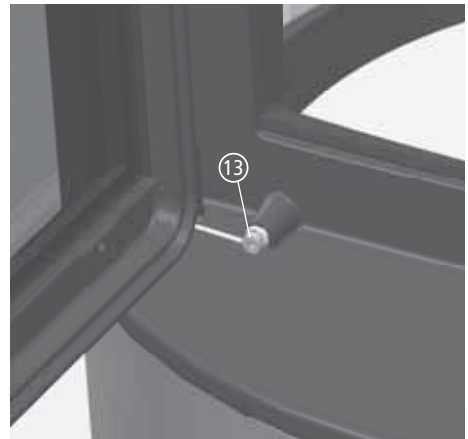
Abb. 3.13 gespannte Türfeder
