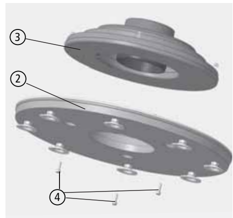
Abb. 3.17 Drehkonsole mit Grundplatte und Oberteil
