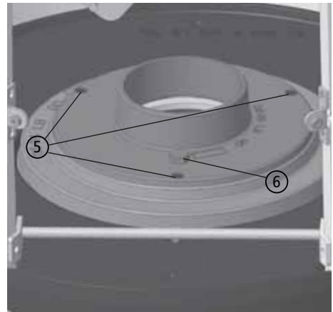
Abb. 3.26 Drehkonsolen-Oberteil montieren
