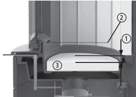
Abb. 4.7 Aschebett, Ascheniveau
