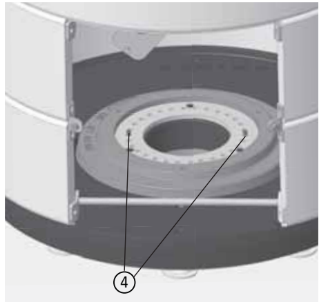
Abb. 3.24 Anschlag-Stifte, Einstellen des linken und rechten Endanschlags
